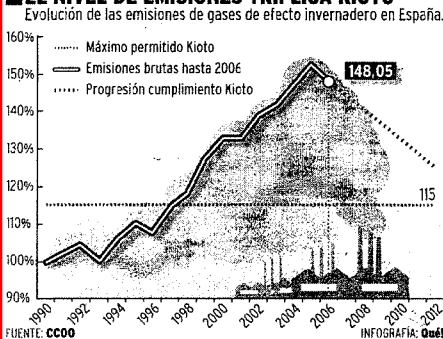
El nivel de emisiones de España se sitúa aún muy lejos de lo que le permite el Protocolo de Kioto.
